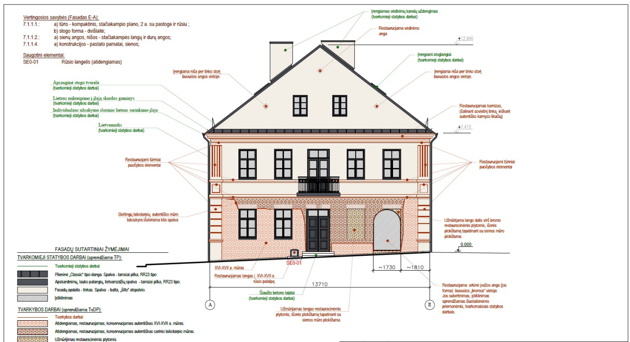
Vazos namo R. fasado sprendinys. Iš techninio projekto.
